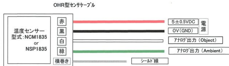
SST-NCM1835 型センサー
