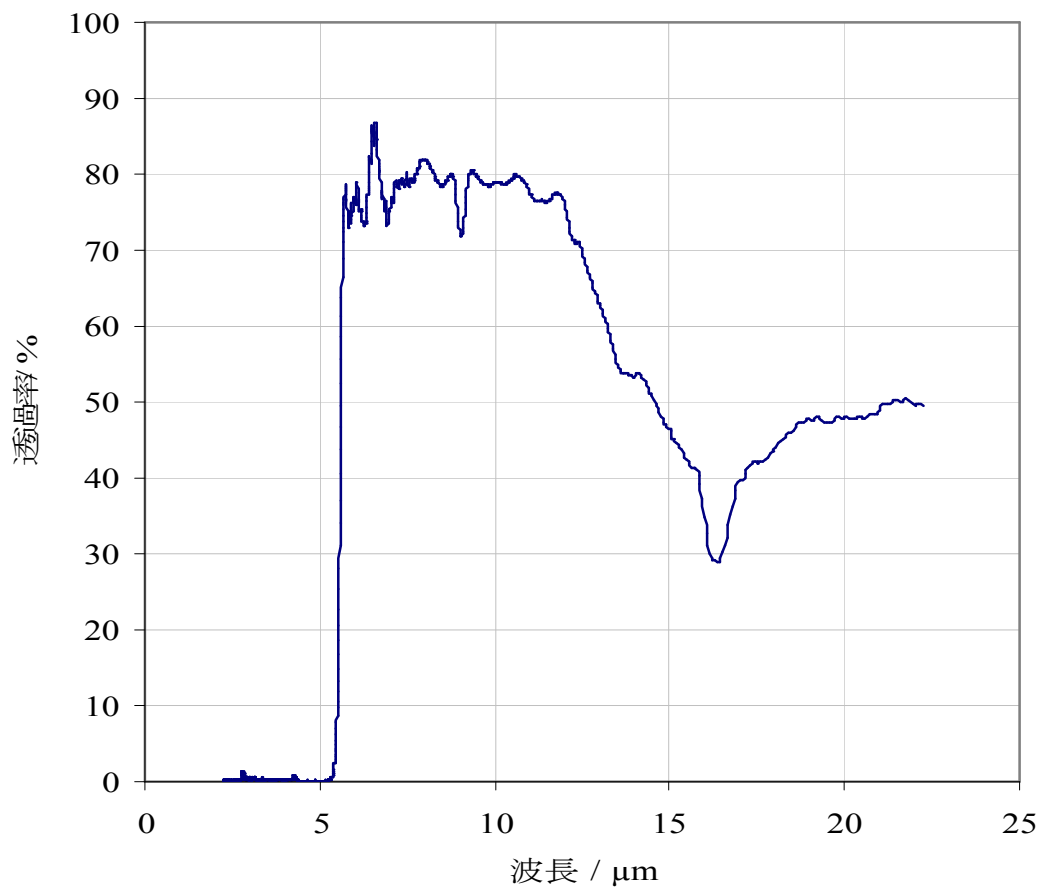
透過特性 5.5 \mu m フィルター (typ)
