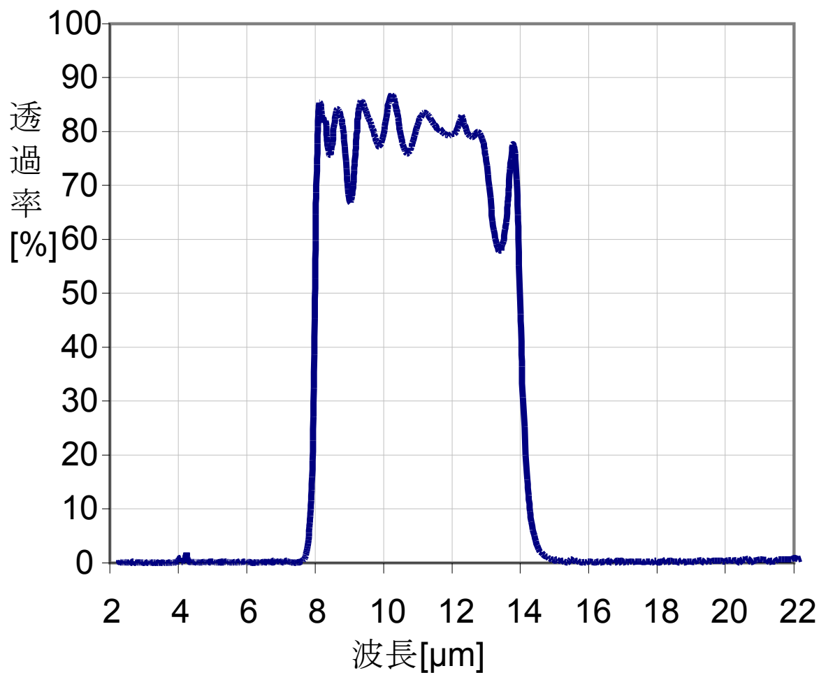
透過特性 8-14 \mu m フィルター (typ)
