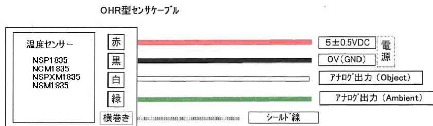
SST-NSPXS1835 型センサー
